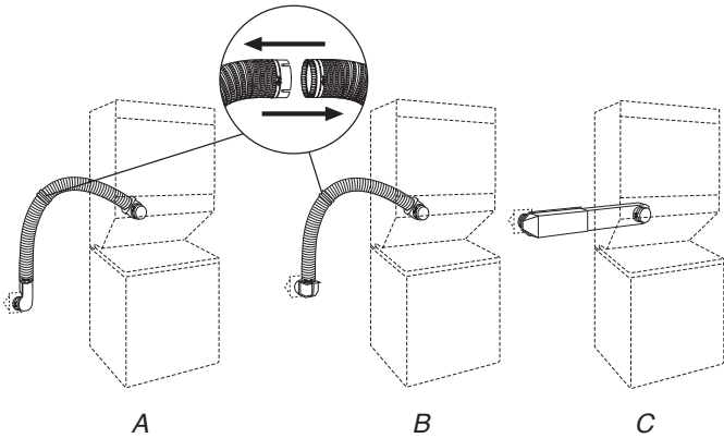
A. Système dévié avec coudes classiques B. Système dévié avec un double coude et un coude classique C. Système d'évacuation avec un périscope (dégagement de 2" [51 mm])
