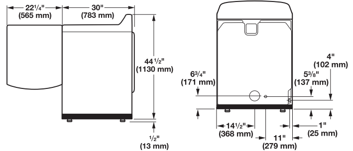
Vue latérale
