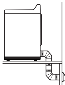
Installation du système d'évacuation en résidence mobile
