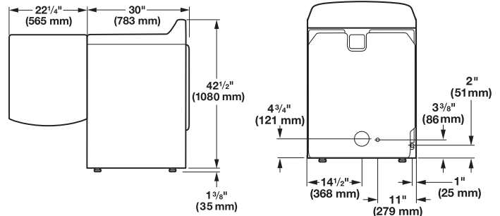
Vue latérale
