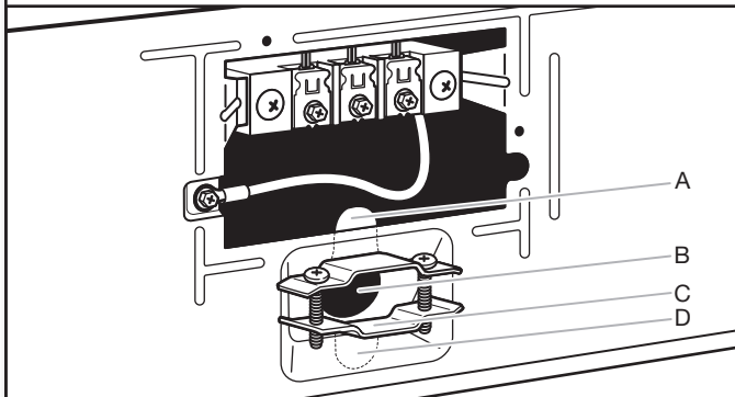
Contacto de 4 hilos (Tipo NEMA 14-30R)
