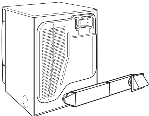
Instalación de periscopio
