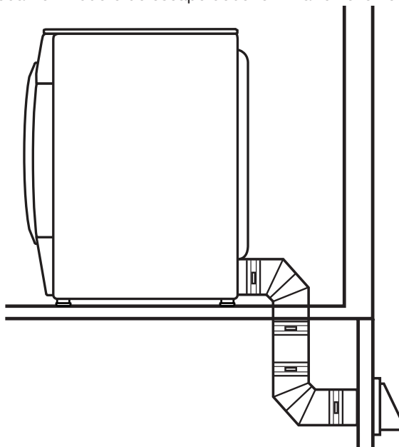
Instalación con ventilación por la parte inferior
