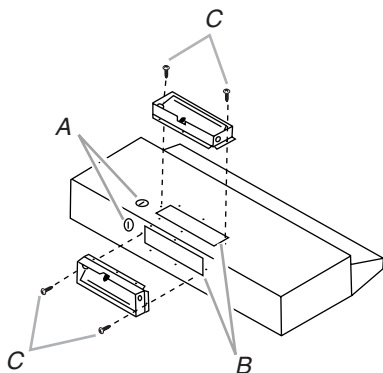
A. Opercules arrachables pour passage du câble d'alimentation B. Opercules arrachables pour circuit d'évacuation C. Vis de tôle n° 8B
