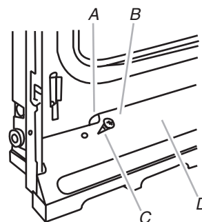
A. Ouverture du châssis du four B. Onglet de l'évent C. Vis n°8-18 de 3/8" D. Évent du four
