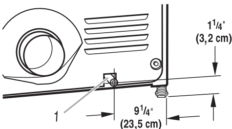
1. Tuyau NPT de la sècheuse de \frac{3}{8} po
