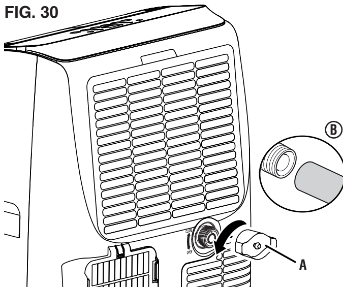
A - Tapón de drenaje superior B - Conexión de la manguera de drenaje
