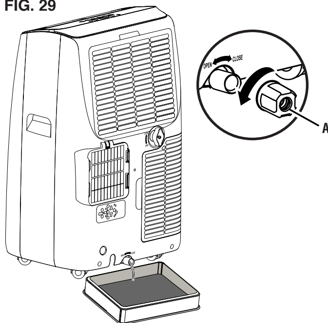
A - Tapón de drenaje inferior
