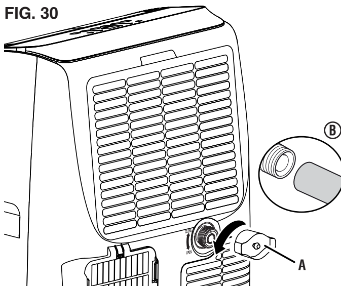
A - Bouchon de vidange supérieur
