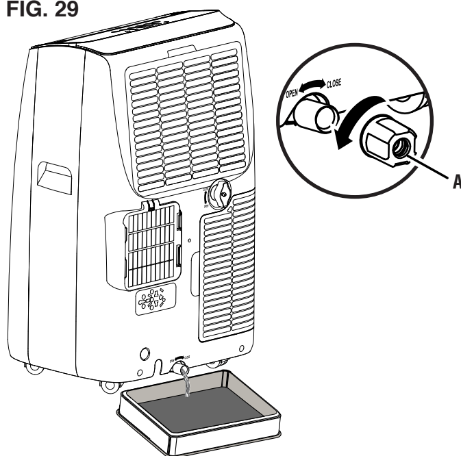
A - Bouchon de vidange inférieur
