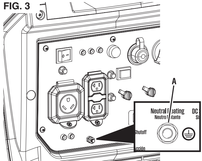
A - Terminal de tierra
