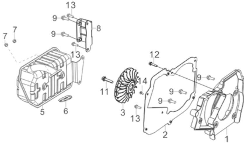
FIG. 11. MUFFLER ASSEMBLY
