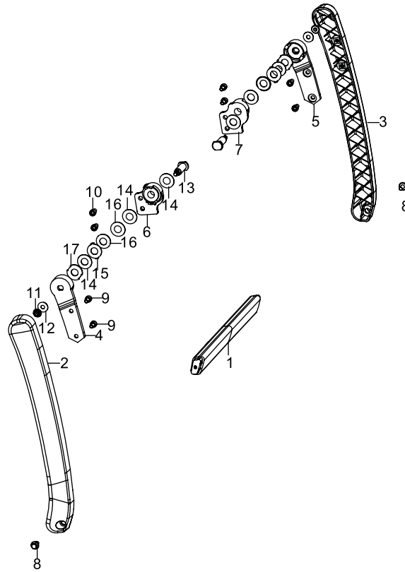
Fig. 15 - Handle
