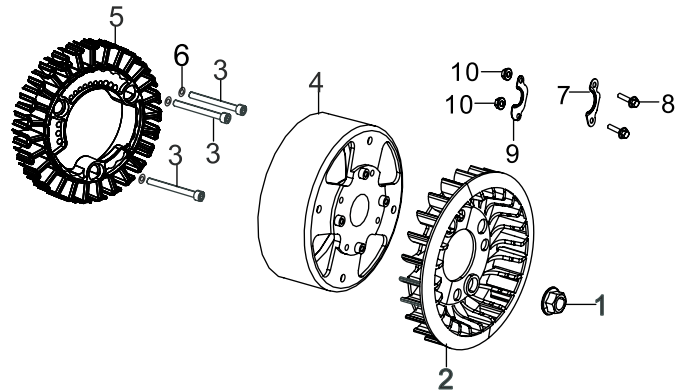
Fig. 9 - Impeller, Alternator
