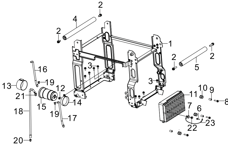
Fig. 13 - Frame
