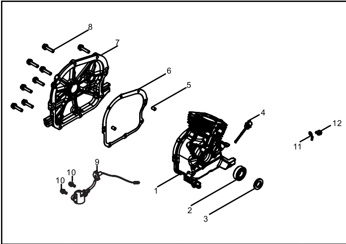
Fig. 1 - Crankcase
