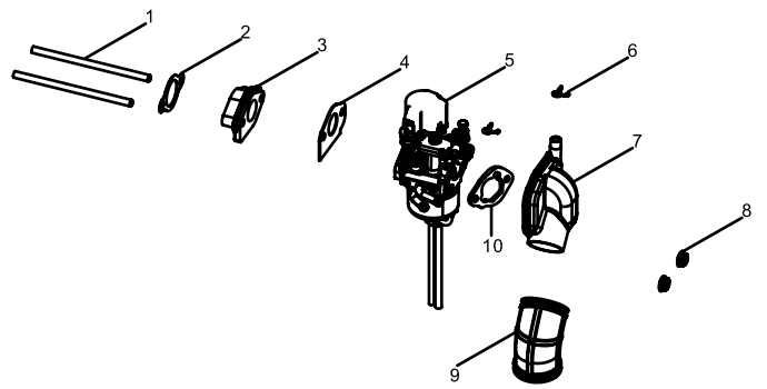
Fig. 6 - Carburetor
