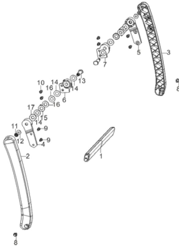
Fig. 15 - Handle
