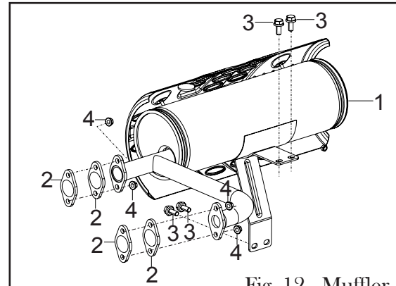
Fig. 12 - Muffler
