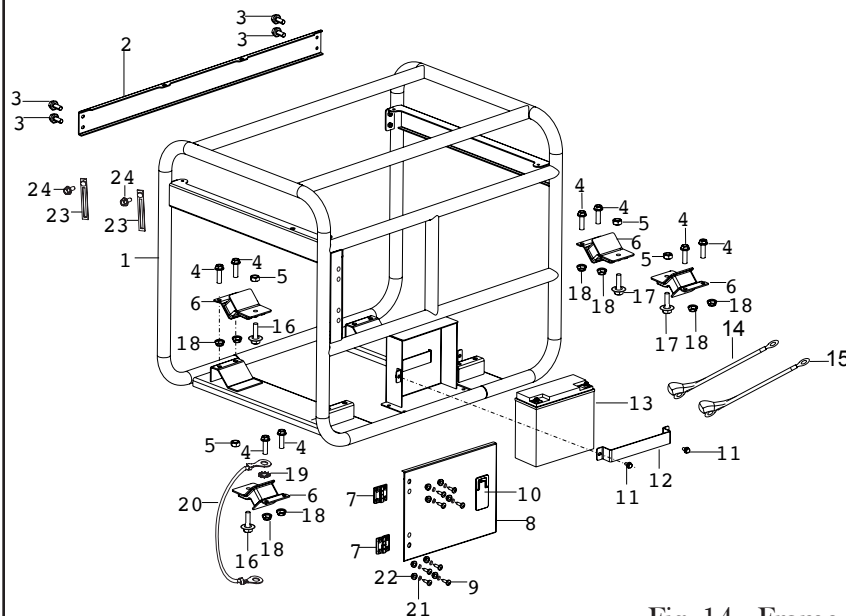
Fig. 14 - Frame
