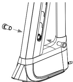
Adapter C Adaptateurs d'axe traversant 15x100
