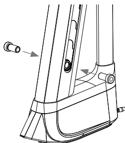
Adapter B 12x100 스크루액슬 어댑터
