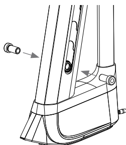
Adapter D 15x110 스크루액슬 어댑터
