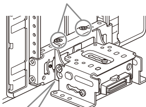
Tornillos instalados previamente
