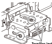
Tornillos instalados previamente
