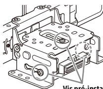
Vis pré-installées
