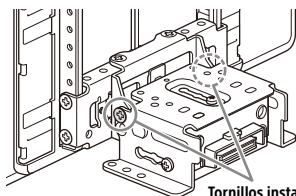
Tornillos instalados previamente
