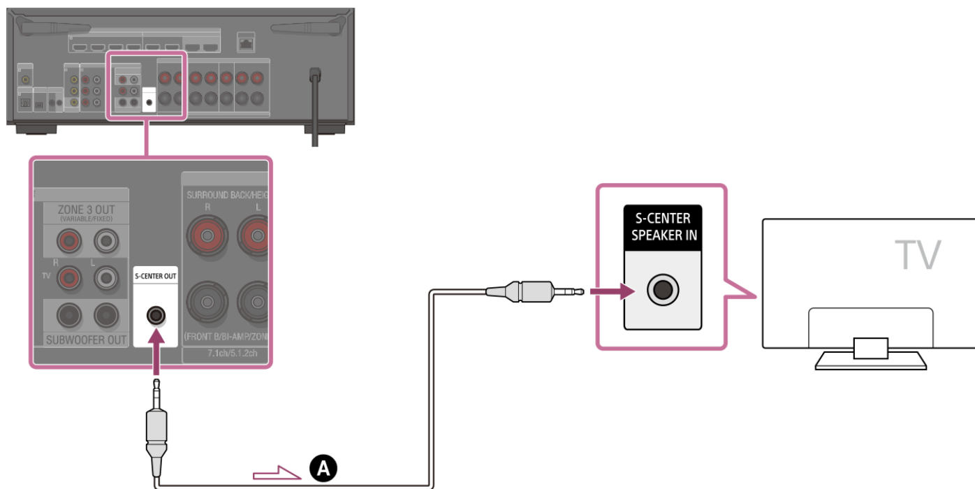
A Câble audio stéréo mini-fiche tripolaire (non fourni)
