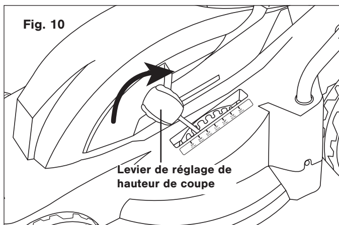
Les 7 positions du réglage de la hauteur de coupe :
