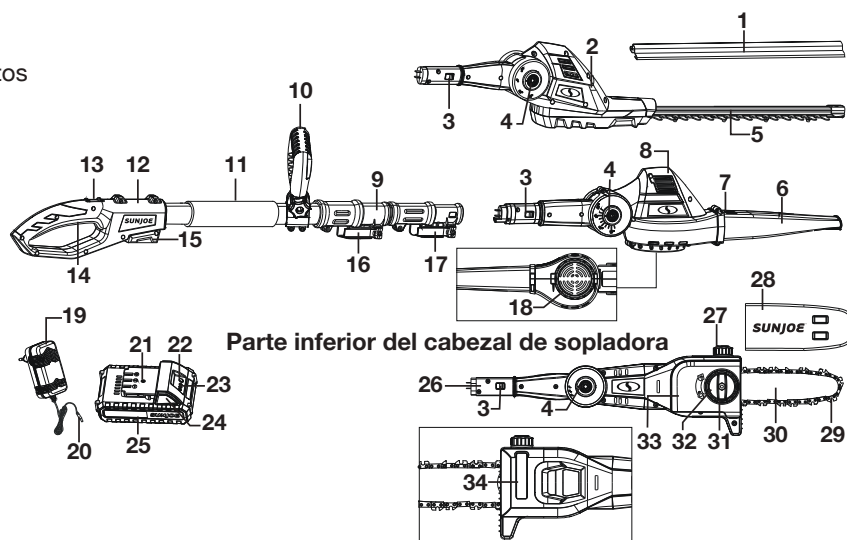
Reverso del cabezal de motosierra
