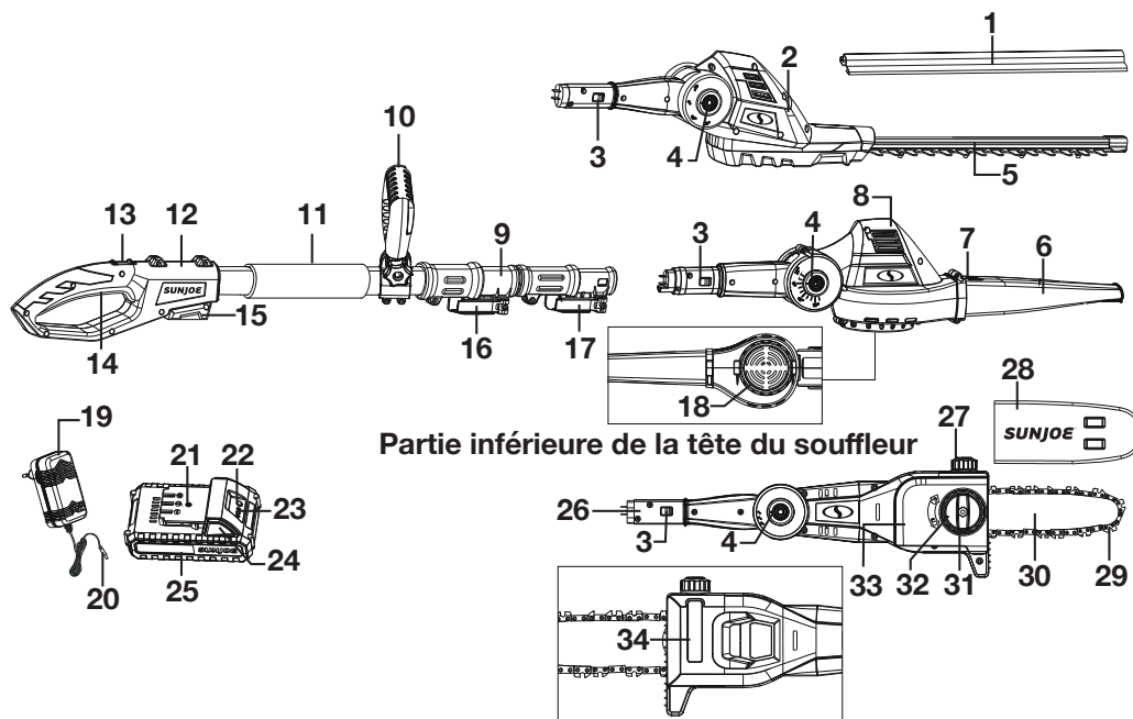
Arrière de la tête porte-scie à chaîne
