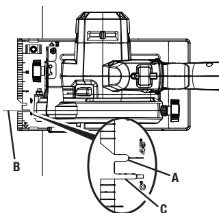
Fig. 15 TOP VIEW OF SAW (VUE SUPÉRIEURE DE SCIE, VISTA SUPERIOR DE LA SIERRA)
