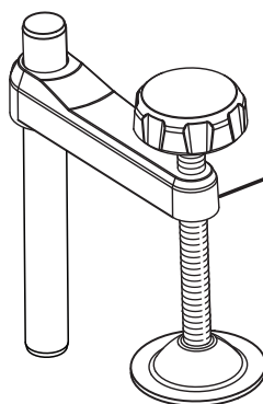
PRENSA DE TRABAJO
