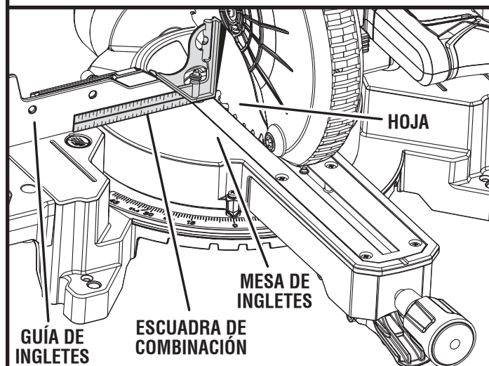
VISTA DE LA HOJA FUERA DE ESCUADRA CON LA MESA DE INGLETES; SE REQUIEREN AJUSTES Fig. 24
