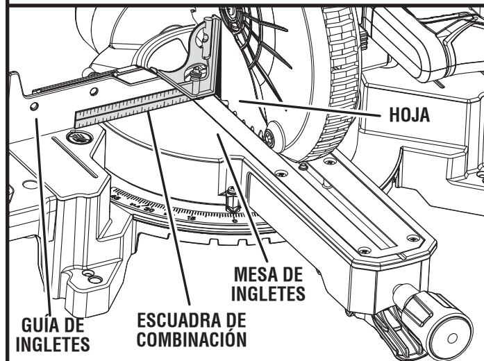
VISTA DE LA HOJA FUERA DE ESCUADRA CON LA MESA DE INGLETES; SE REQUIEREN AJUSTES Fig. 25
