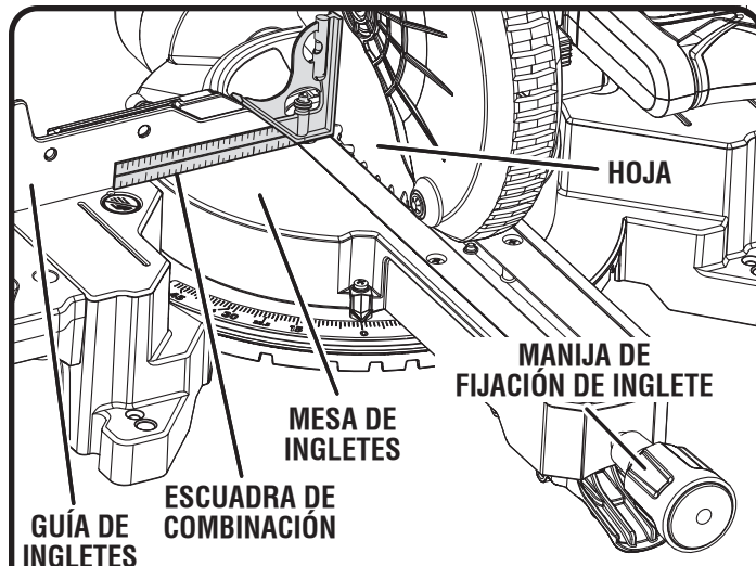
VISTA CORRECTA DE LA HOJA A ESCUADRA CON LA MESA DE INGLETES Fig. 23
