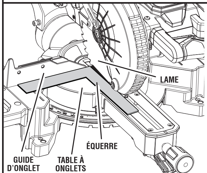
VUE DE LA LAME PAS D'ÉQUERRE AVEC LE GUIDE, DES RÉGLAGES SONT NÉCESSAIRES
