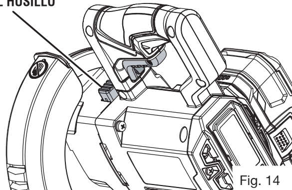
BOTÓN DEL SEGURO DEL HUSILLO
