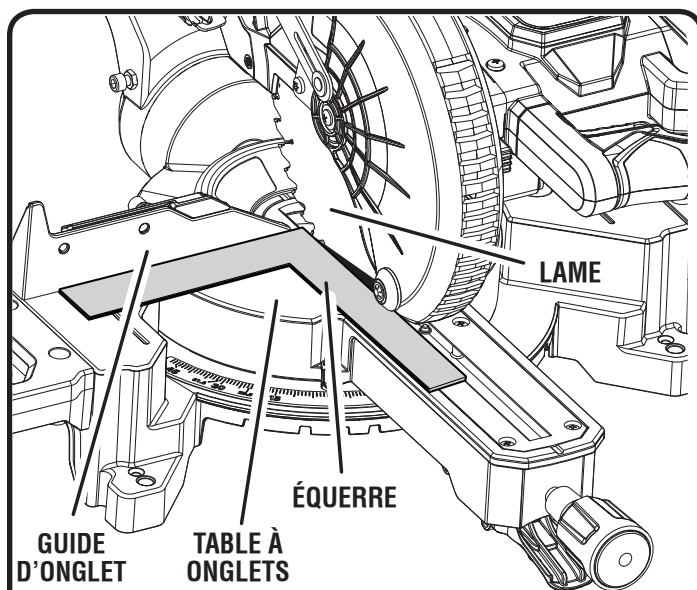
VUE DE LA LAME PAS D'ÉQUERRE AVEC LE GUIDE, DES RÉGLAGES SONT NÉCESSAIRES
