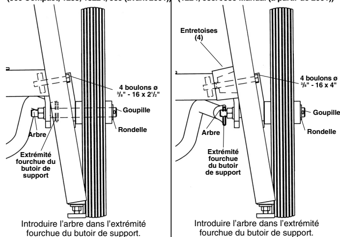
Figure 3 – Largeur d'assise du support (détail de la Figure 2)
