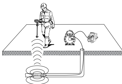
Figura 19 – Localizar a Sonda Reel
