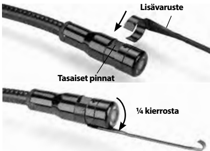
Kuva 8 – Lisävarusteen asentaminen
