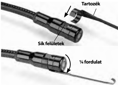
8. ábra – Tartozék csatlakoztatása
