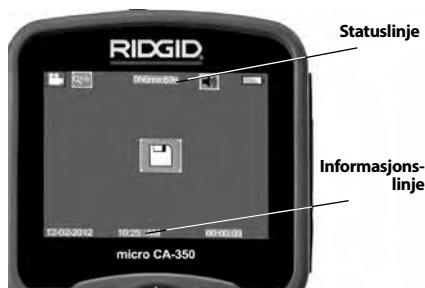
Figur 12 – Direktebilde
