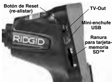
Figura 4 – Puertos del lado izquierdo
