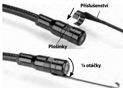
Obrázek 8 – Instalace příslušenství
