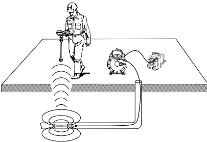
Slika 19 - Lociranje namatajuće sonde
