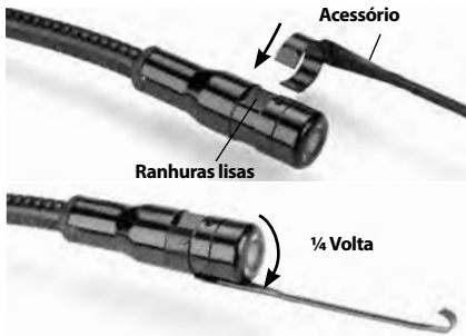
Figura 8 - Instalar um Acessório
