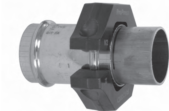
Figure 12B – Positionnement de bague ProPress sur raccord
