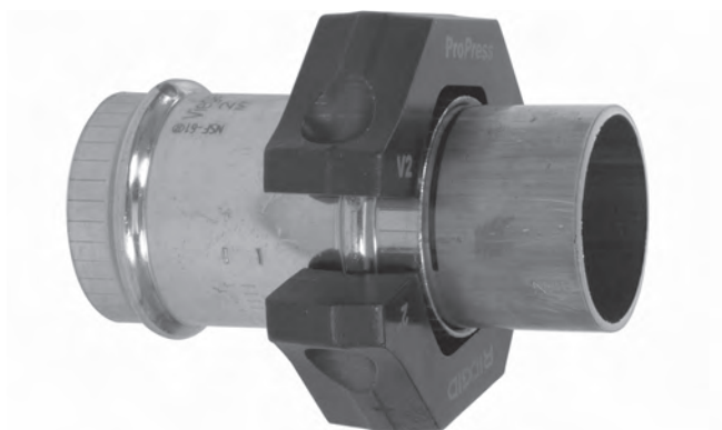
Figura 12B – Montaje del aro ProPress alrededor del acoplamiento
