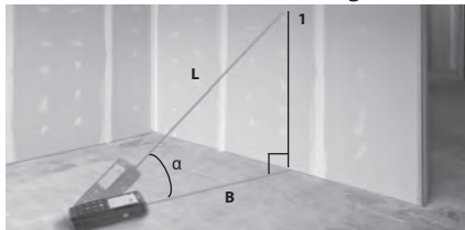
Abbildung 12 – Indirekte horizontale Entfernung
