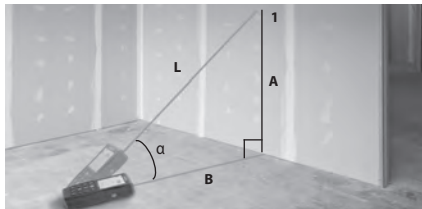
Abbildung 11 – Indirekte horizontale und vertikale Entfernung
