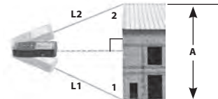
Abbildung 14 – Indirekte vertikale Entfernung unter Verwendung von zwei Punkten (Gesamthöhe)
