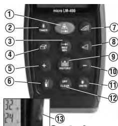
Figura 3 – Controles del telémetro láser micro LM-400
