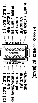
12MW DEUTSCH DT RECEPTACLE CONNECTOR (DTP-4-279) WEDGE LOCK (W12P)
