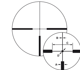
Podświetlana siatka celownicza nr 4 z kropką
