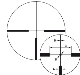
Retícula núm. 4 de IL con punto
