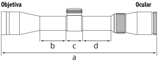
As letras de a a d no diagrama acima se referem aos comprimentos (a) a (d), mostrados na tabela de especificações.
