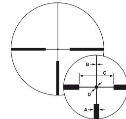
Megvilágított 4-es célkeresztponttal
