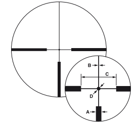
Beleuchtetes Absehen 4 mit Punkt
