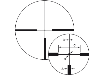
Подсвеченная визирная сетка #4 с точкой
