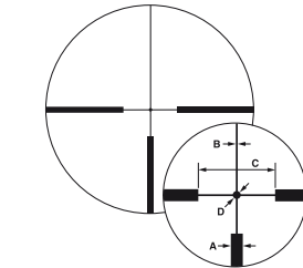
Osvětlený nitkový kříž číslo 4 s tečkou
