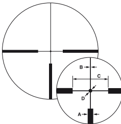
IL-ristikko nro 4, jossa on piste
