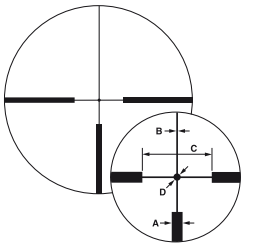
Reticulul IL #4 cu punct
