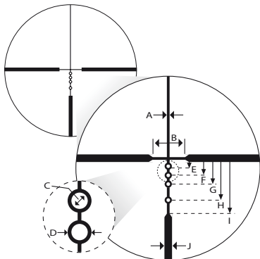
Réticule BDC 150
