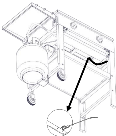
quemador principal
