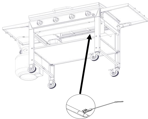
Quemador Principal
