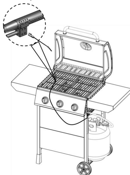
Brûleur Principal
