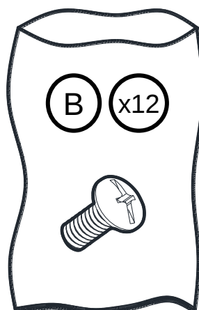
Truss Head Screw Traversenkopfschraube Truss hovedskrue Fackverkshuvudskruv Vis cruciforme Tornillo de cabeza ovalada 5/32 - 32 x 2/5"
