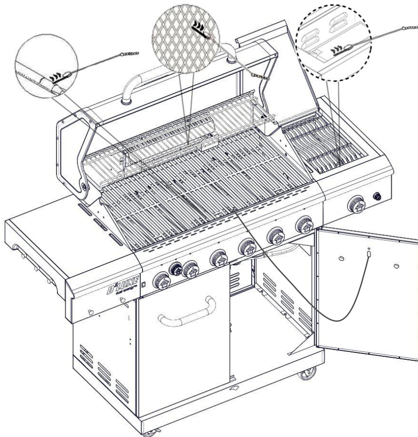
Quemador principal
