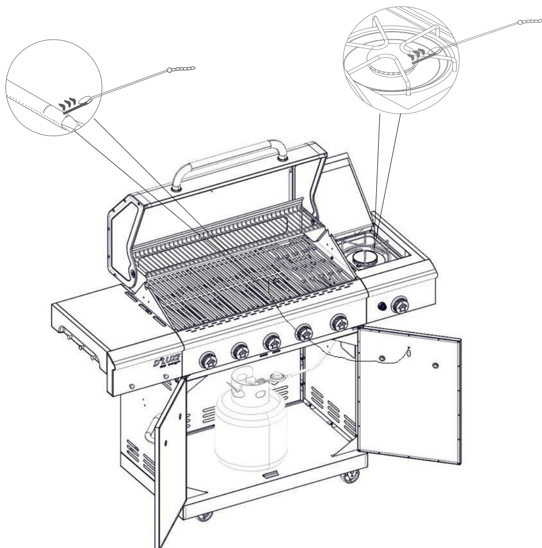
Brûleur principal
