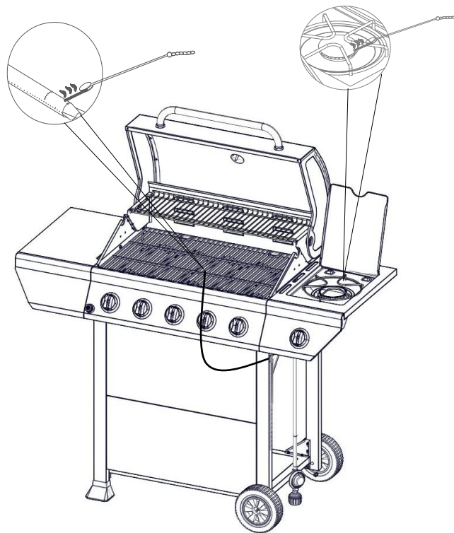
brûleur principal
