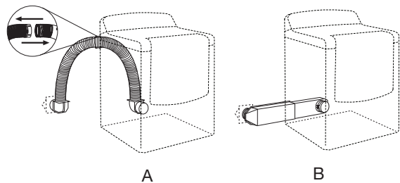
A. Instalación por la parte superior (también está disponible con un codo de desviación) B. Instalación del periscopio
