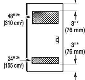
Puerta de clóset con orificios de ventilación
