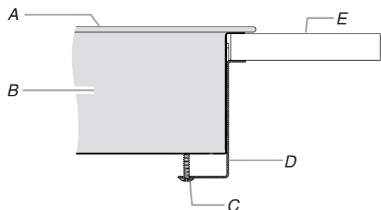
A. Table de cuisson B. Base de la table de cuisson C. Vis de fixation de bride de 2" (5,1 cm) D. Bride de fixation (dépassant suffisamment de la base de la table de cuisson pour permettre l'installation des vis de fixation) E. Plan de travail
