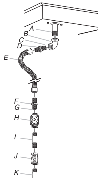
A. Entrée de la tubulure B. Coude de 3/8" C. Utiliser un composé d'étanchéité des tuyauteries. D. Raccord d'adaptation (avec filetage mâle 3/8") E. Raccord flexible (à passer dans le mur entre les placards) F. Raccord d'adaptation (avec filetage mâle 3/8") G. Utiliser un composé d'étanchéité des tuyauteries. H. Détendeur de l'appareil (fourni) I. Tuyau de gaz de 1/2" ou 3/4" J. Robinet d'arrêt manuel K. Tuyau de gaz de 1/2" ou 3/4"
