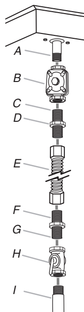
A. Entrée de la tubulure B. Détendeur C. Utiliser un composé d'étanchéité des tuyauteries. D. Raccord d'adaptation (avec filetage mâle 1/2") E. Raccord flexible F. Raccord d'adaptation G. Utiliser un composé d'étanchéité des tuyauteries. H. Robinet d'arrêt manuel I. Tuyau de gaz de 1/2" ou 3/4"
