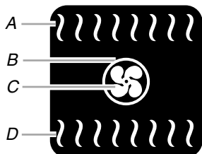
A. Élément de cuisson au gril B. Élément de cuisson C. Ventilateur de convection D. Élément de cuisson au four
