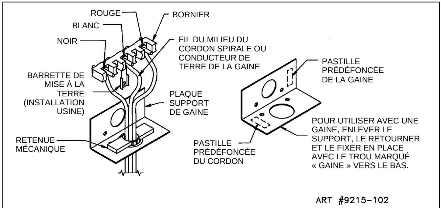
FIGURE 7 INSTALLATION ACCEPTABLE - FICHE À TROIS FILS
