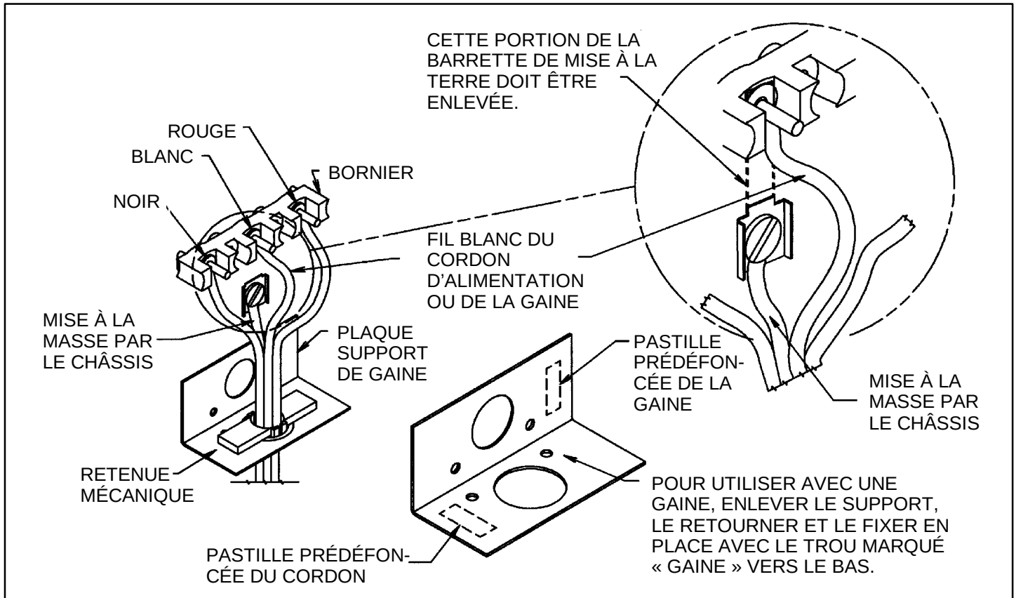
FIGURE 8 INSTALLATION ACCEPTABLE - FICHE À QUATRE FILS
