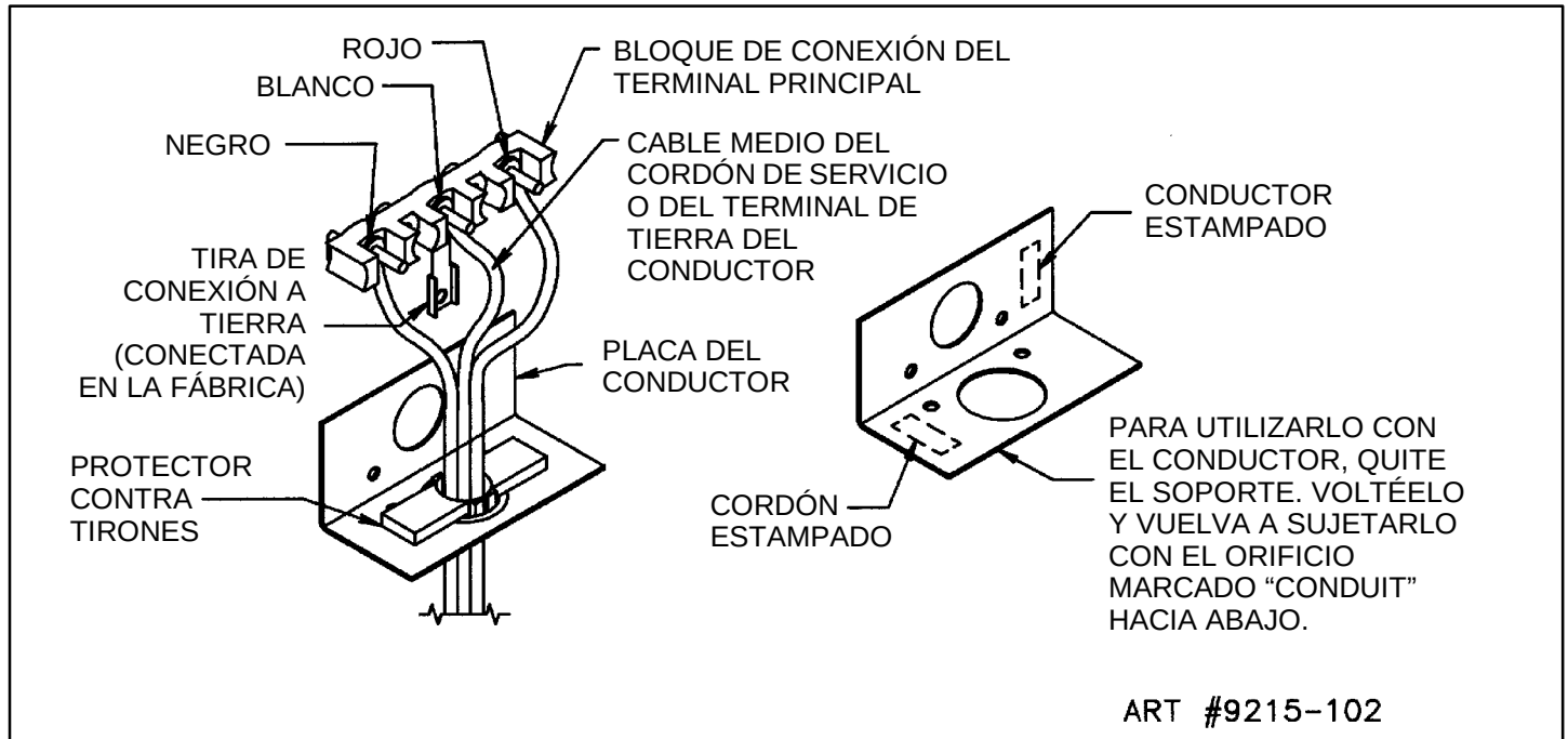
FIGURA 7 INSTALACIÓN ACEPTADA DEL ENCHUFE DE 3 CABLES
