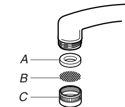
A. Arandela B. Filtro C. Portafiltro o aereador
