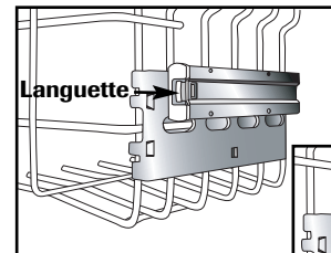
Butée avec languette de sûreté
