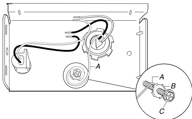
A. Conducteur de liaison à la terre vert B. Rondelle C. Vis verte de liaison à la terre
