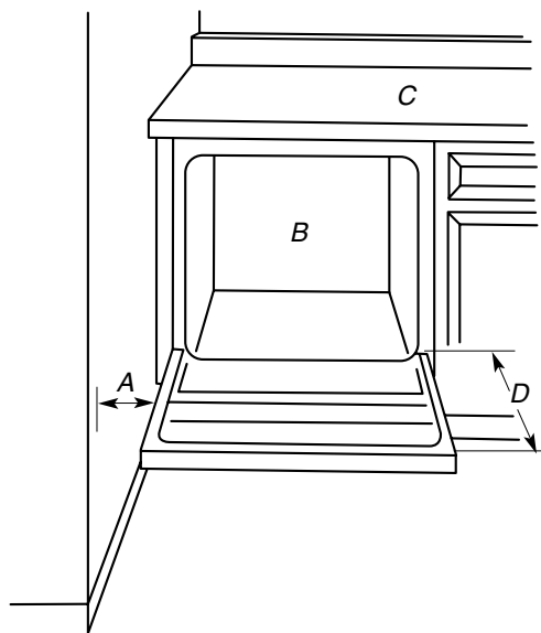
A. Dégagement minimal de 2" (5,1 cm) pour l'ouverture de la porte B. Lave-vaisselle
