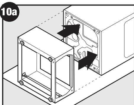
10a Position riser./Positionnez le socle./Coloque el pedestal en posición.
