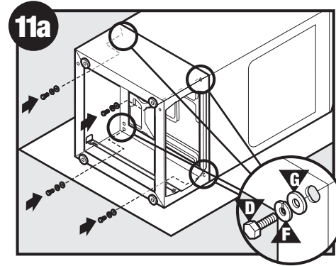
11a Secure riser to appliance with bolts and washers. Go to step 13./Fixez le socle à l'appareil avec les vis et les rondelles. Référez-vous à l'étape 13./Fije el pedestal al electrodoméstico con pernos y arandelas. Vaya al paso 13.
