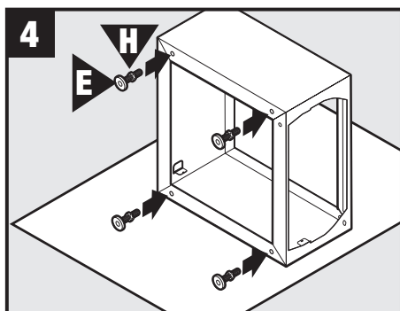
4 Attach leveler legs./Installez les pieds de mise à niveau./Instale las patas niveladoras.
