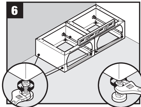
6 Level riser(s) and lock in leg heights./Mettez le ou les socles de niveau et verrouillez les pieds./Nivele el(los) pedestal(es) y bloquee la altura de las patas.
