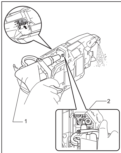
► 1. Pistola sacudidora de aire 2. Guía
