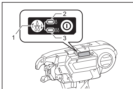
► 1. Botón de conmutación de modo 2. Modo de accionamiento simple 3. Modo de accionamiento continuo
