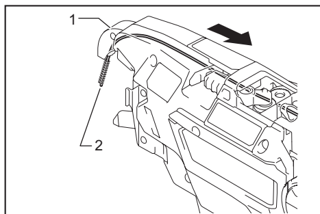
► 1. Brazo de la herramienta 2. Cepillo de alambre
