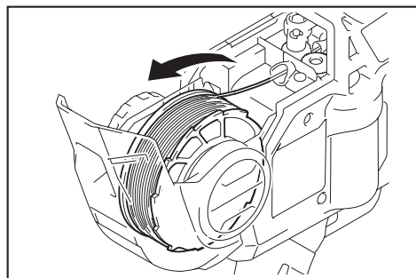
► 1. Engranaje 2. Ruta del alambre 3. Alambre
