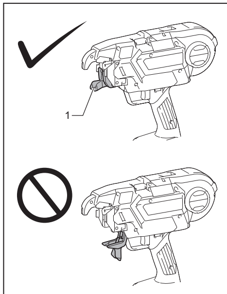
► 1. Guía de volutas
