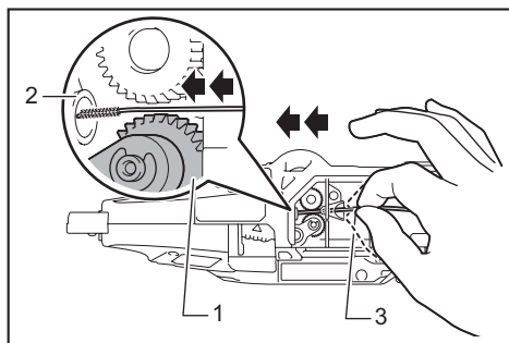
► 1. Engranaje 2. Guía 3. Cepillo de alambre
