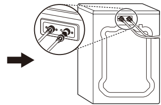
Raccordement des tuyaux d'alimentation
