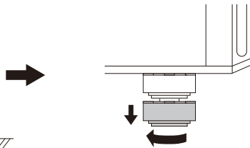
Nivellement de la laveuse
