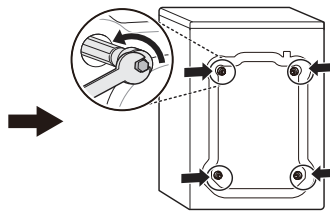
Déballage et retrait des boulons d'expédition
