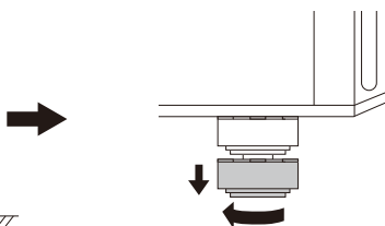
Nivelado de la lavadora
