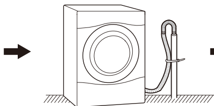
Raccordement du tuyau de vidange
