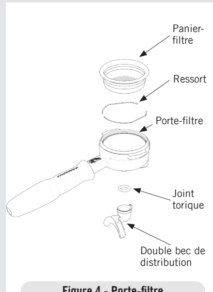
Figure 4 - Porte-filtre
