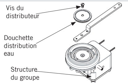
Figure 7 - Groupe Café
