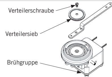
Abbildung 7 - Brühgruppensystem
