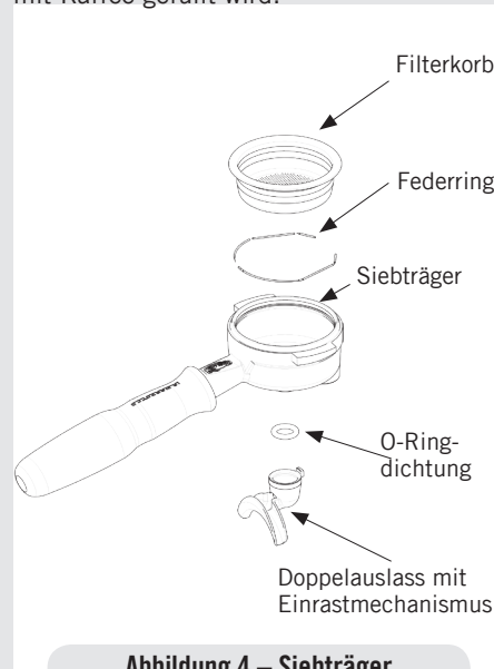
Abbildung 4 – Siebträger
