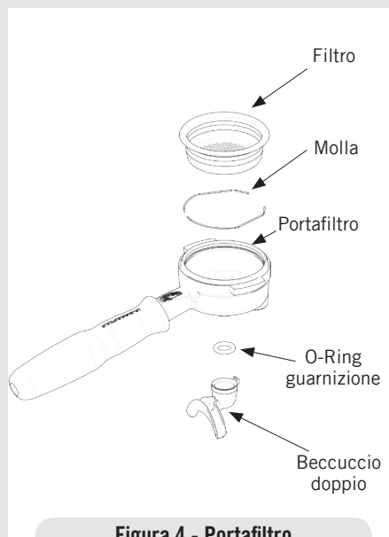
Figura 4 - Portafiltro
