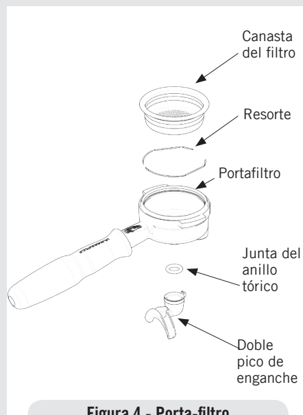
Figura 4 - Porta-filtro
