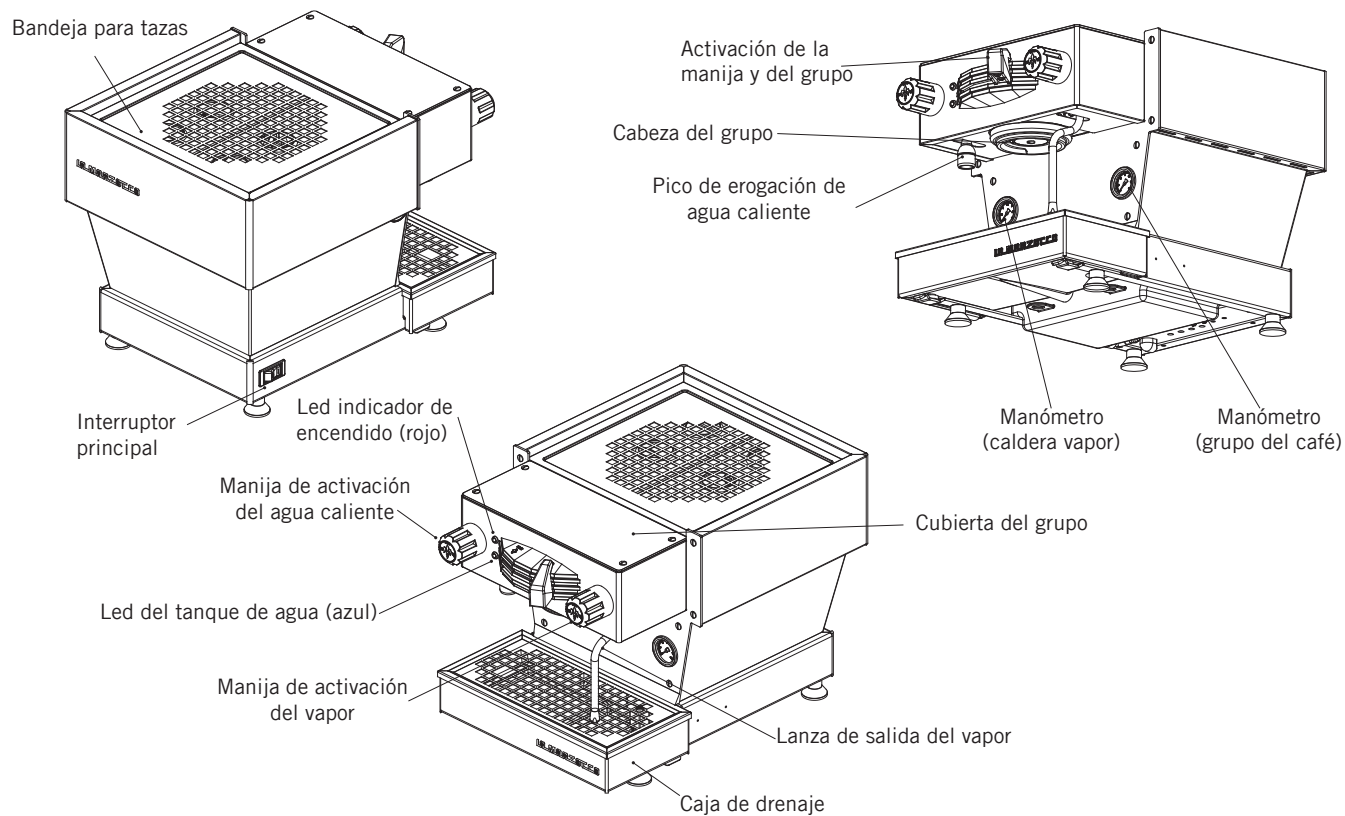
Figura 1 - Descripción de la Máquina
