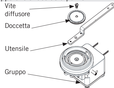
Figura 7 - Gruppo Caffè
