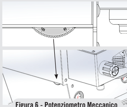
Figura 6 - Potenzimetro Meccanico
