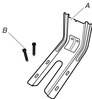
A. Bride antibascullement B. Vis de montage n° 12 x 1 \frac{5}{8} "
