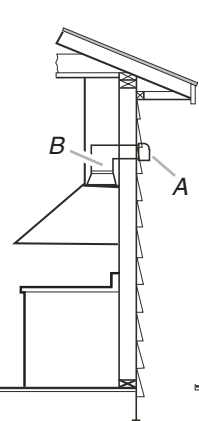
A. Bouche de décharge murale B. Conduit rond 6" (15,2 cm)
