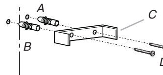
A. Chevilles d'ancrage de 8 x 40 mm B. Axe central sur le mur C. Bride de support du cache-conduit D. Vis de 5 x 45 mm
