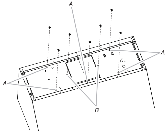
A. Emplacement des écrous à emboîter pour le système à deux ventilateurs (quantité 5) B. Emplacement des écrous à emboîter pour le système à un seul ventilateur (quantité 2)
