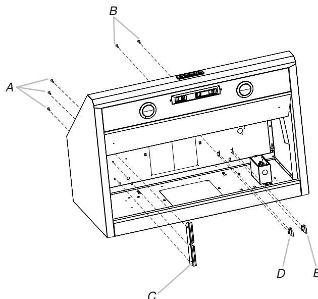
A. 3 vis 4,2 x 8 mm pour le support de montage du moteur B. 2 vis 4,2 x 8 mm pour la languette à ressort du moteur C. Support de montage du moteur D. Languette à ressort du moteur (emplacement pour système à un seul ventilateur) E. Languette à ressort du moteur (emplacement pour système à deux ventilateurs)
