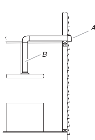
A. Bouche de décharge murale B. Conduit rond, dia. 10" (25,4 cm)
