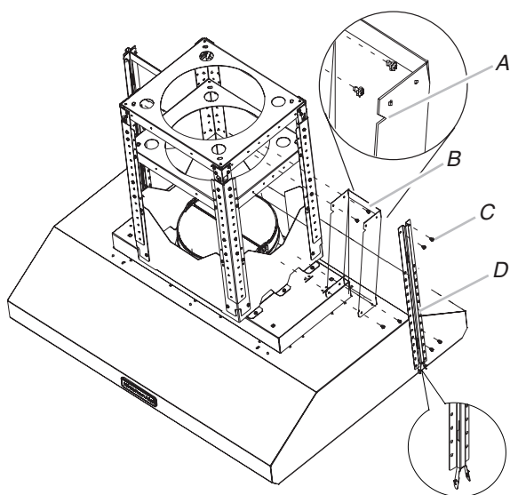
A. Encoche dans le support B. Support C. Vis de 4,2 x 8 mm D. Support du cache-conduit vertical
