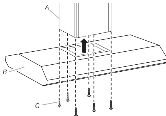
A. Cache-cheminée – section inférieure B. Auvent de la hotte de cuisinière C. 6 vis de 4,2 x 8 mm
