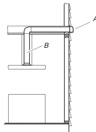
A. Wall cap B. 10" (25.4 cm) round vent
