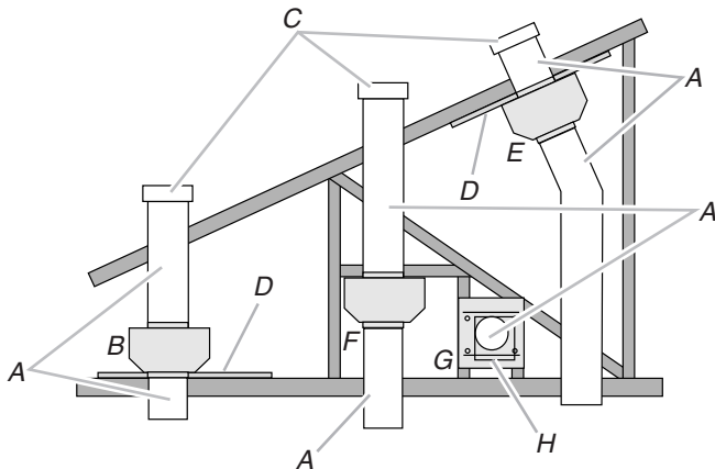
A. Conduit rond de 10" (25,4 cm) B. Fixation au dessus des solives de plafond C. Bouches de décharge par le toit D. Contreplaqué (facultatif pour certaines configurations d'installation) E. Fixation sur le dessous des chevrons du toit F. Fixation des traverses de cadre de châssis aux fermes G. Conduit horizontal; fixation des traverses de cadre de châssis aux fermes H. Bouche de décharge murale
